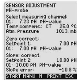
Корректировка датчика
